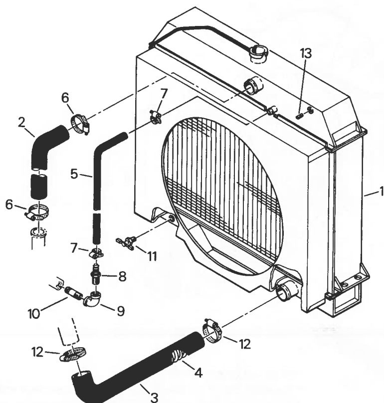
Cat 3406
